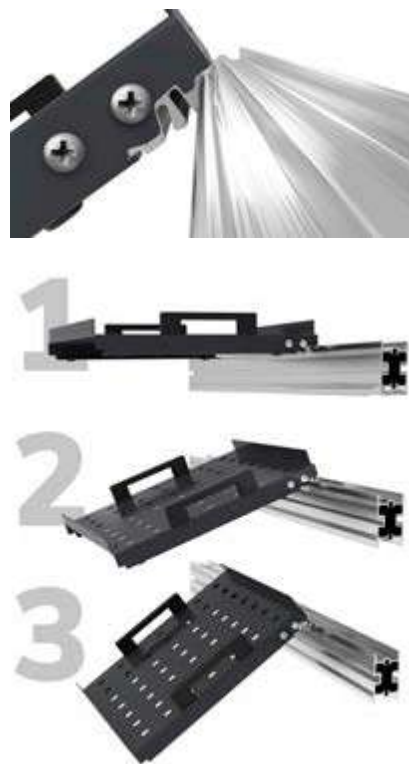
SOSTEGNO DA TAVOLO PER VASSOIO PIKPAD 5S SHADOW TOOL BOX
