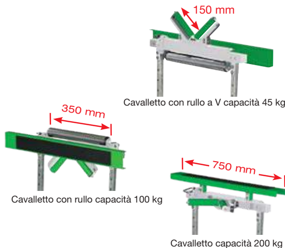
Cavalletto capacità 200 kg
