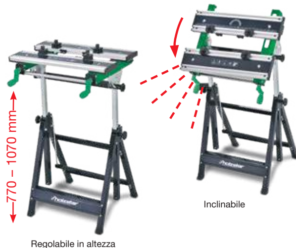
Regolabile in altezza
